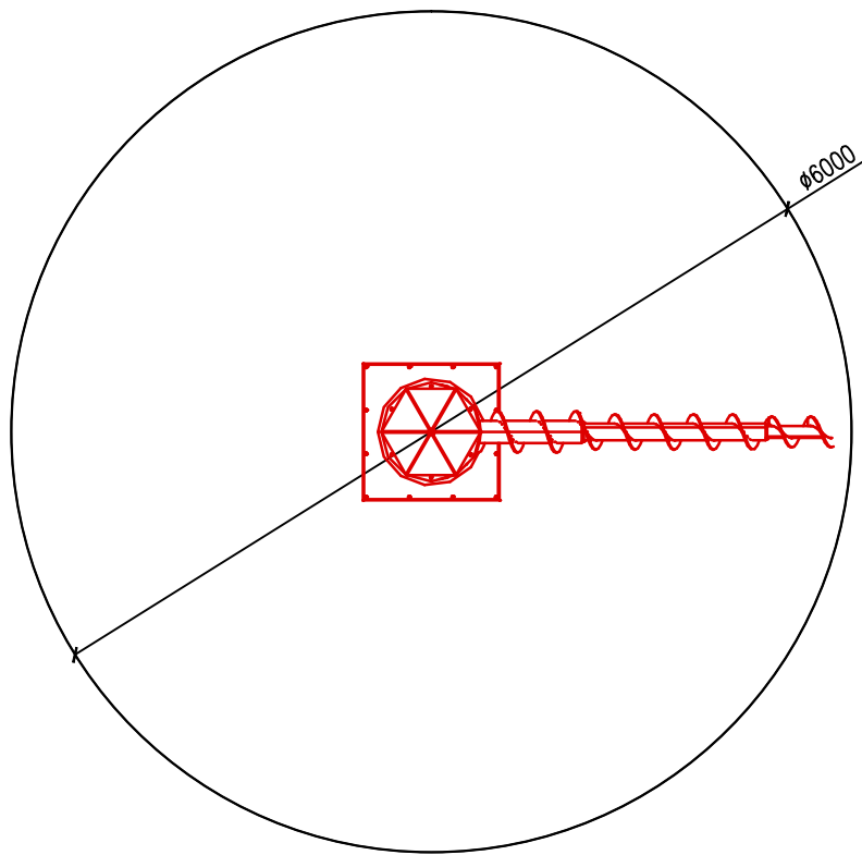
Розріз А-А
